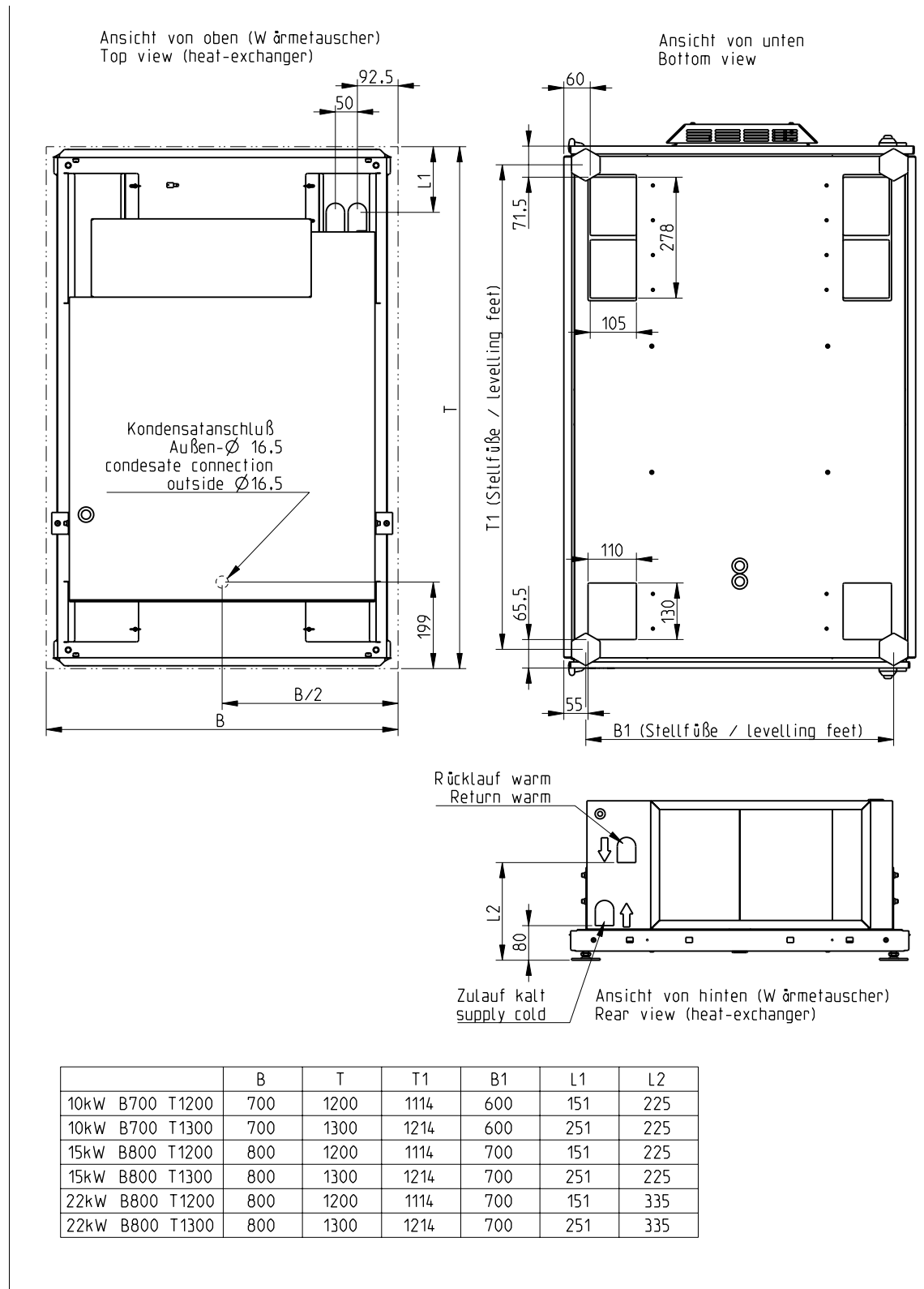
Abmessungen Bodenplatte / Öffnungen / Anschlüsse 12- 17 - 25 / 35 kW
